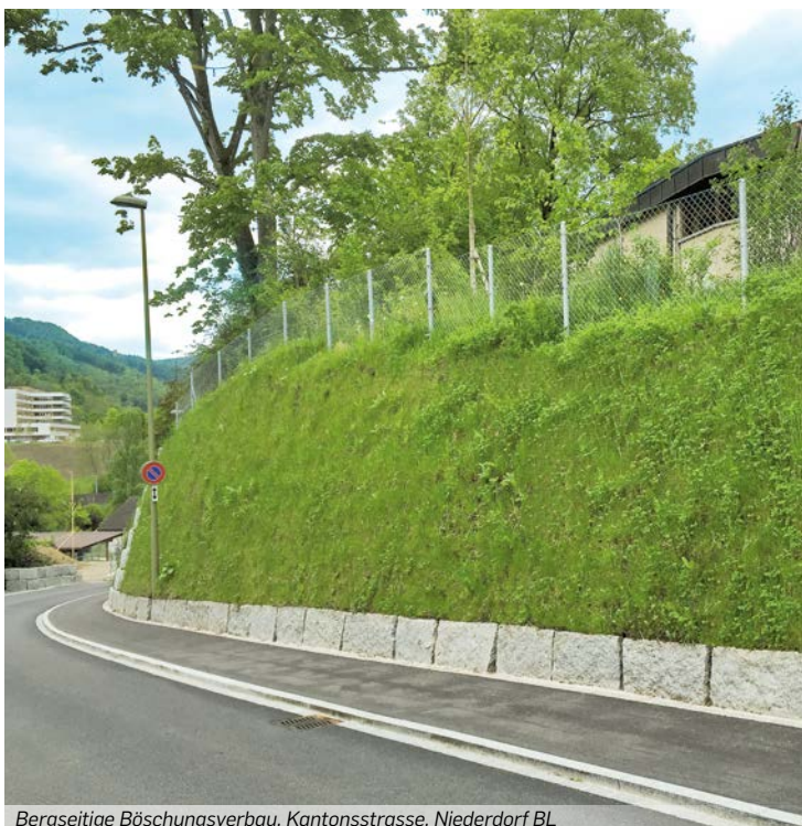
Bergseitige Böschungsverbau, Kantonsstrasse, Niederdorf BL
